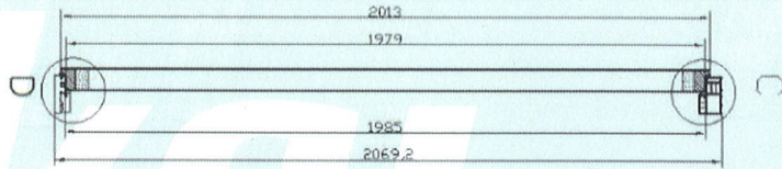
수직단면상세도
