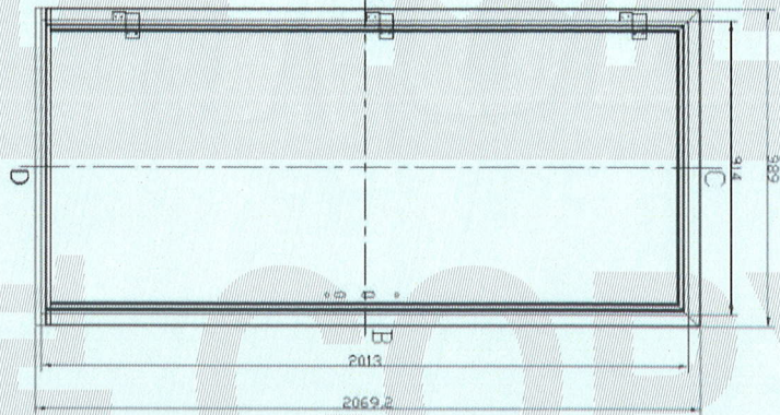
인면도
